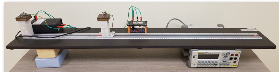
Urządzenie do pomiaru rezystancji włókienniczych wyrobów liniowych
